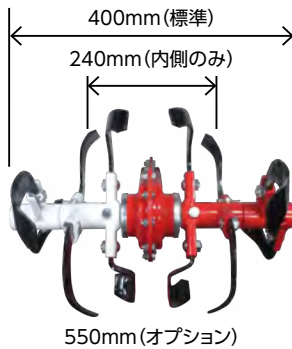
中耕刃受作業幅
