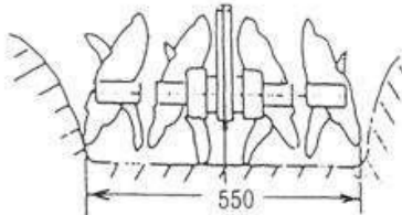
デスクローター4速（両排）コードNo. C46-1503-000
