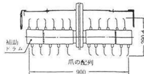
補助ドラム付の場合
